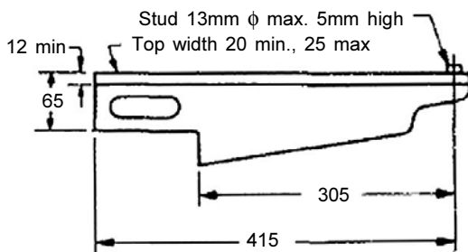
a) Bracket with Lug
