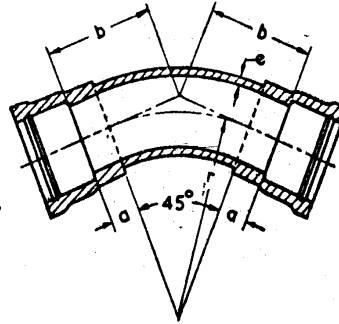
Bend 45°
